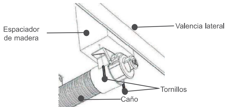
Fig. 16 Conectar la salida del caño al vehículo
