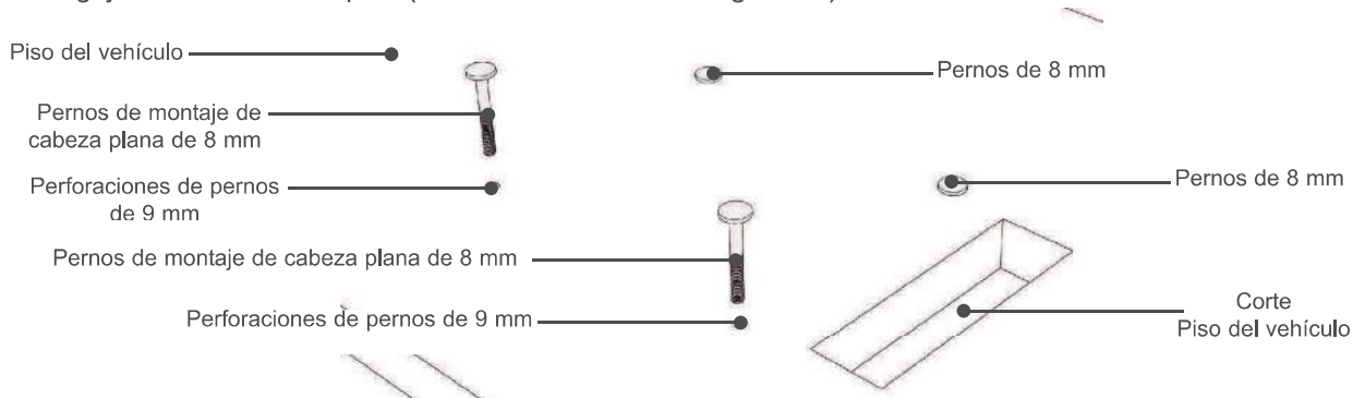
Fig. 10 Fijar pernos de montaje
