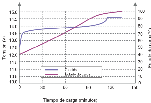
Curvas de estado de carga (0.5C, 25° C)
